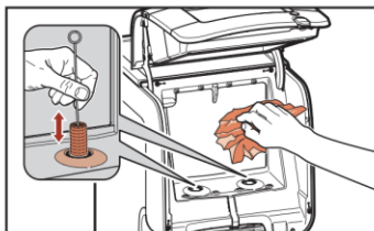
Mynd 5.9 - Hreinsun kærlírmis
