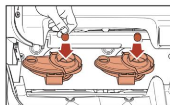
Mynd 5.4 - Ísetning Rinza hreinsitaflna
